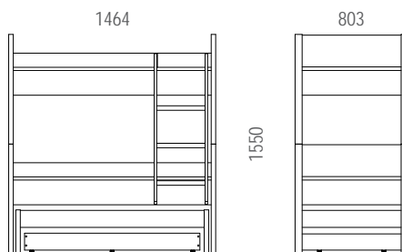
LASTEN KERROSSÄNKY, kaksiosainen
